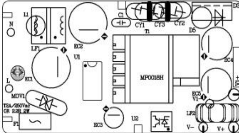
TOP OVERLAY
